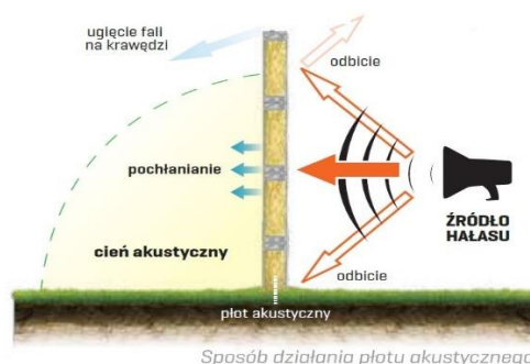
Sposób działania plotu akustycznego
